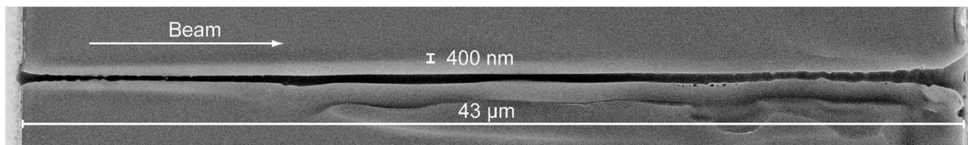
Figure 2. Nano-canal percé dans une lame de verre par une impulsion femtoseconde unique, mise en forme de faisceau de Bessel.
