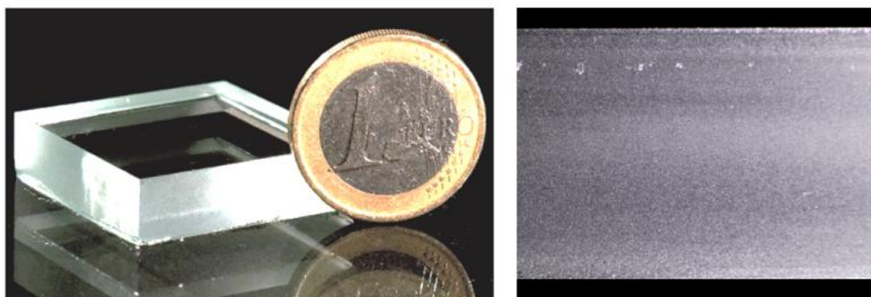
Figure 3. Verre épais découpé par la technique de stealth dicing. L'image de droite présente une vue au microscope d'un verre de 8 mm d'épaisseur après découpe (© Rémi Meyer, FEMTO-ST).
