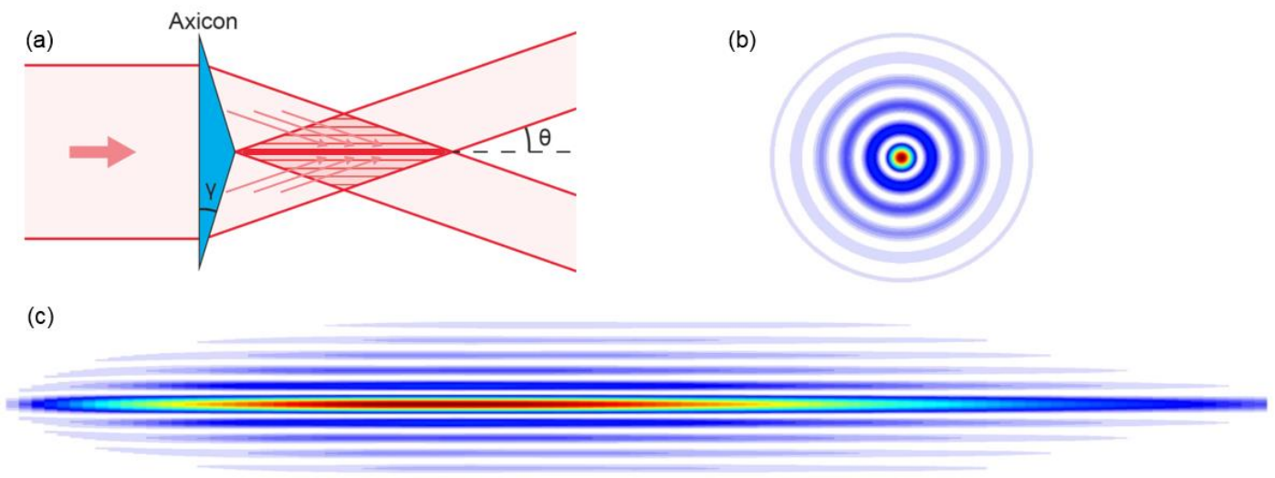
Figure 1. Formation d'un faisceau de Bessel. (a) Ce type de faisceau consiste en un champ d'interférence, par exemple produit via une lentille conique, i.e. , un axicon. Les flèches indiquent la propagation des rayons lumineux, faisant apparaître la structure conique du faisceau. (b) Le profil transverse est formé d'un lobe central intense entouré par des lobes de moindre intensité. Ces lobes sont d'autant plus nombreux que le faisceau est long. (c) La coupe longitudinale de la distribution d'intensité montre que le faisceau est quasiment invariant avec la propagation. En particulier, la dimension du lobe central ne change pas lors de la propagation. Ces propriétés sont également conservées pour des impulsions courtes.
