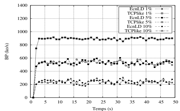
FIGURE 3. EcnLD vs TCPLike pour deux retransmissions Mac.
