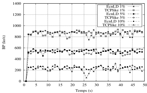
FIGURE 5. EcnLD vs TCPLike pour deux retransmissions Mac et un flux TCP.
