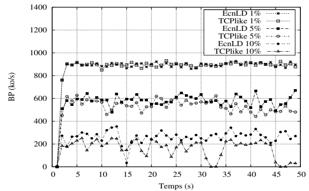
FIGURE 2. EcnLD vs TCPLike pour une retransmission Mac.
