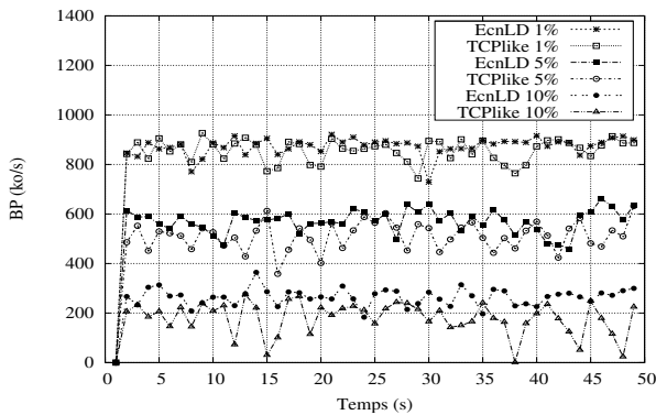
FIGURE 4. EcnLD vs TCPLike pour une retransmission Mac et un flux TCP.
